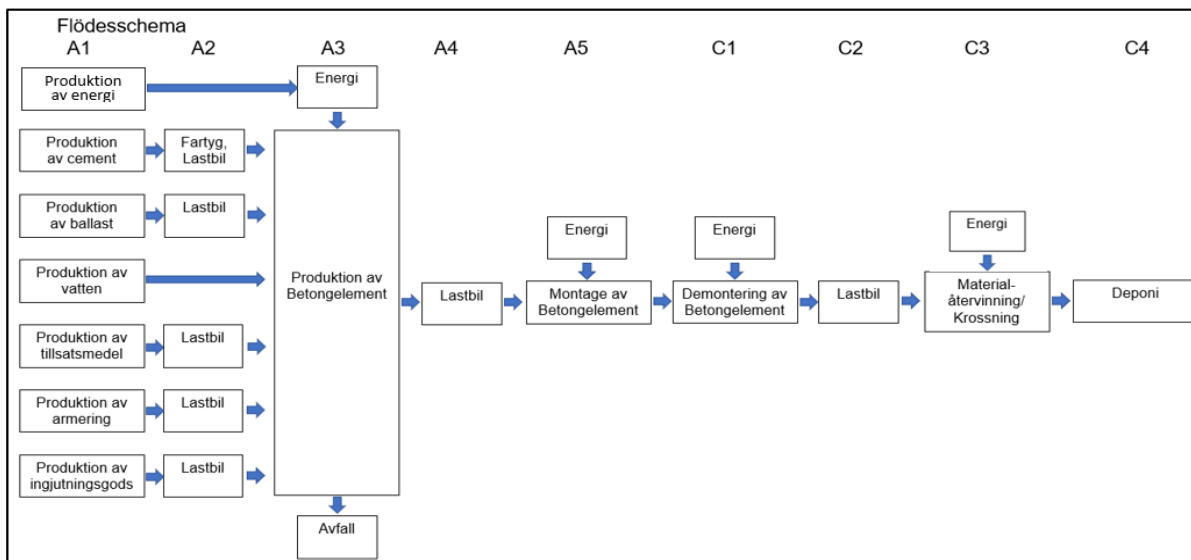
Figur 1. Flödesschema över processer medräknade i livscykel.
